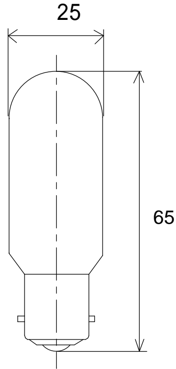
BA15d口金
