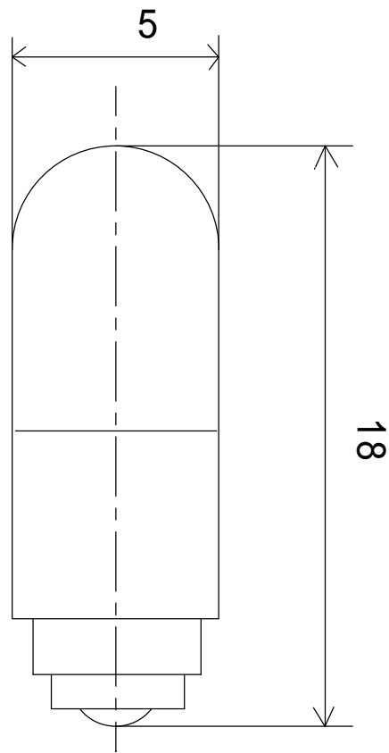
T 5 . 5 段付口金
