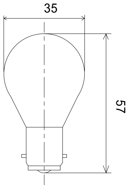
BA15d口金
