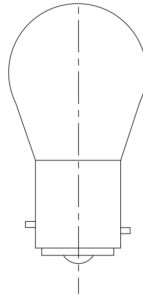
BA15d口金
