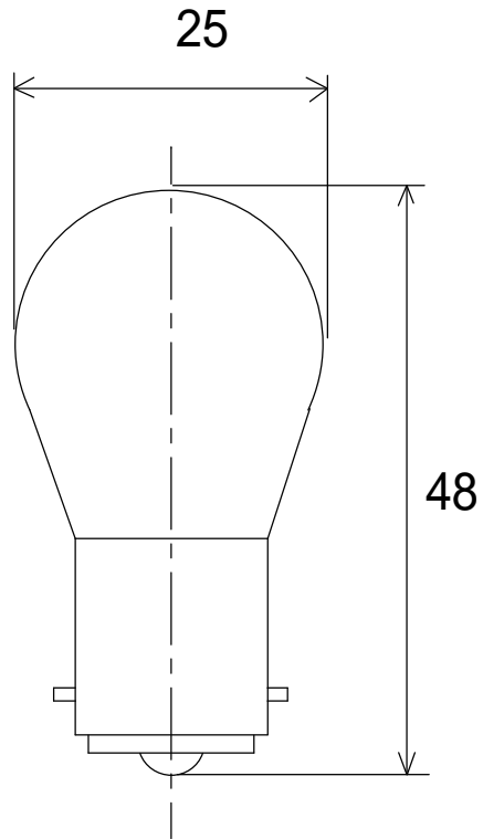
BA15s口金
