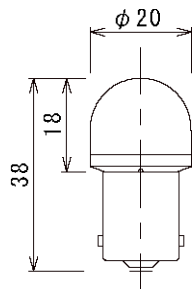
BA 15 s 口金
