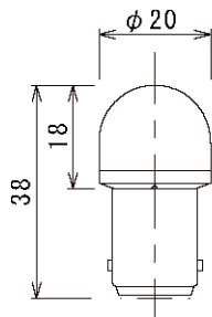
BA 15 d 口金
